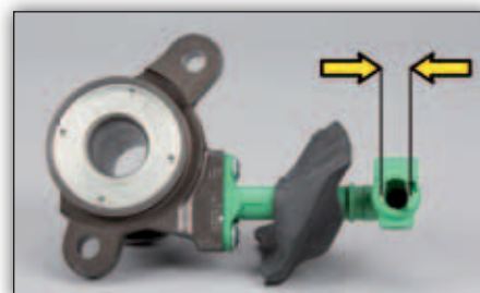
Bild 4: LuK CSC 510 0137 10 Hydraulanslutning 12,2 mm
