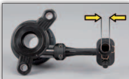
Bild 3: LuK CSC 510 0098 10 Hydraulanslutning 11,7 mm
