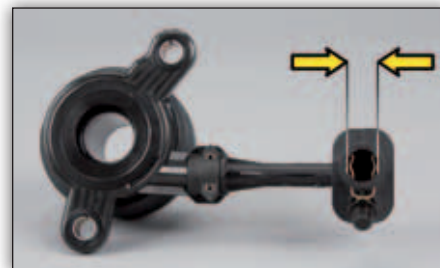
Bild 2: LuK CSC 510 0097 10 Hydraulanslutning 13,3 mm
