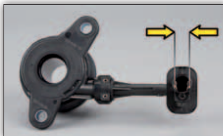
Bild 1: LuK CSC 510 0090 10 Hydraulanslutning 12,2 mm
